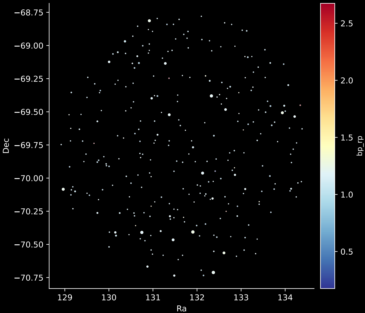
GALAH DR4 Field: [7075] Stars: 281
