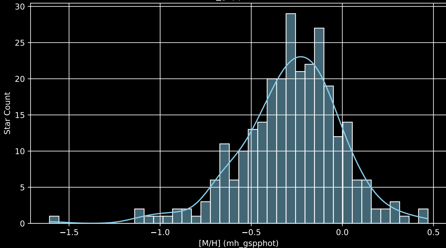
GALAH DR4 Field: [7075] [M/H] (mh_gspphot) (n= 280)
