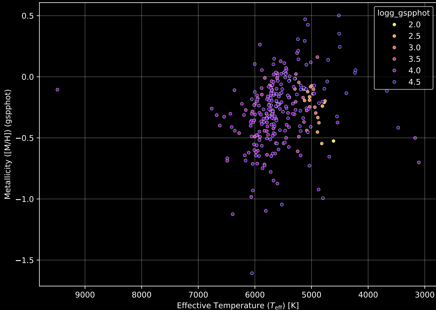
GALAH DR4 Field: [7075] Stellar Population Parameters (n= 281)
