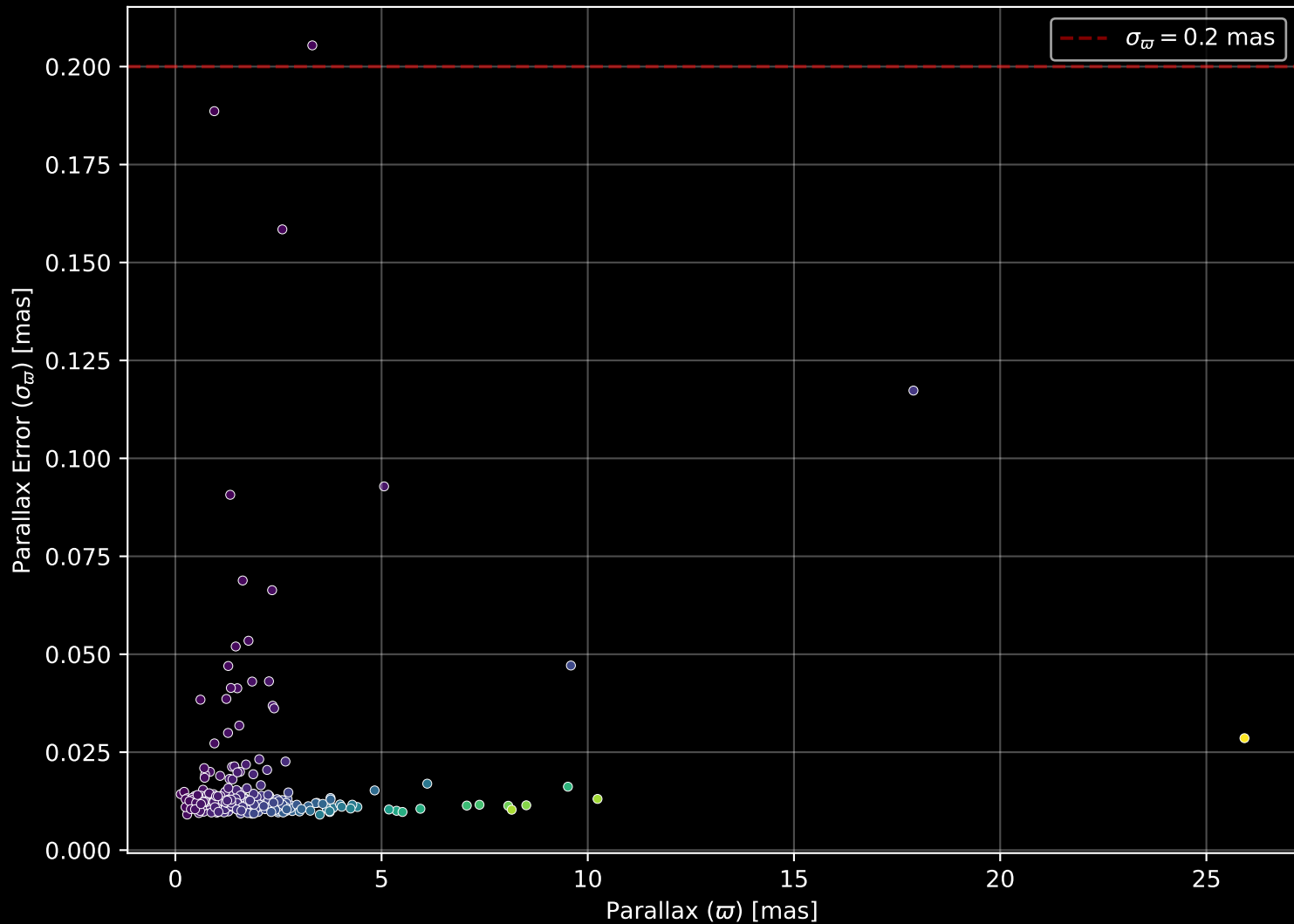
GALAH DR4 Field: [7075] Parallax Quality (n= 281)
